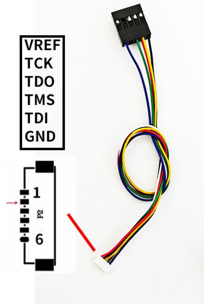
△极简1.25mm 6接口
